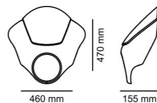
CV10 VARIANTE 1
