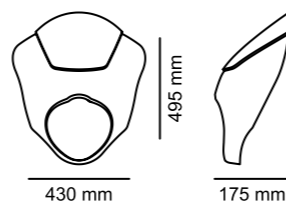
CV10 VARIANTE 2
