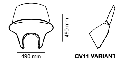
CV11 VARIANTE 1
