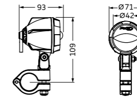
DIMENSIONES
