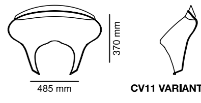
CV11 VARIANTE 2
